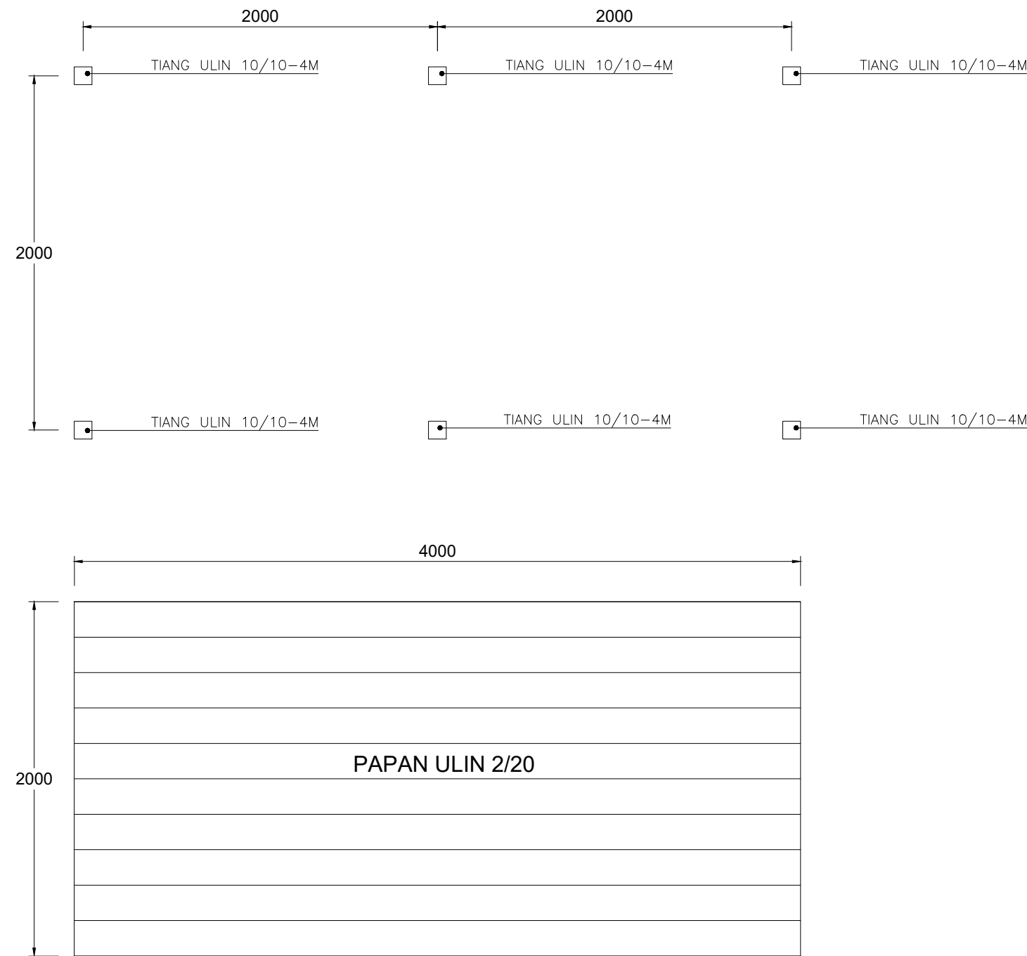
DENAH TITIK PANCANG 1 SKALA 1 : 100 01
