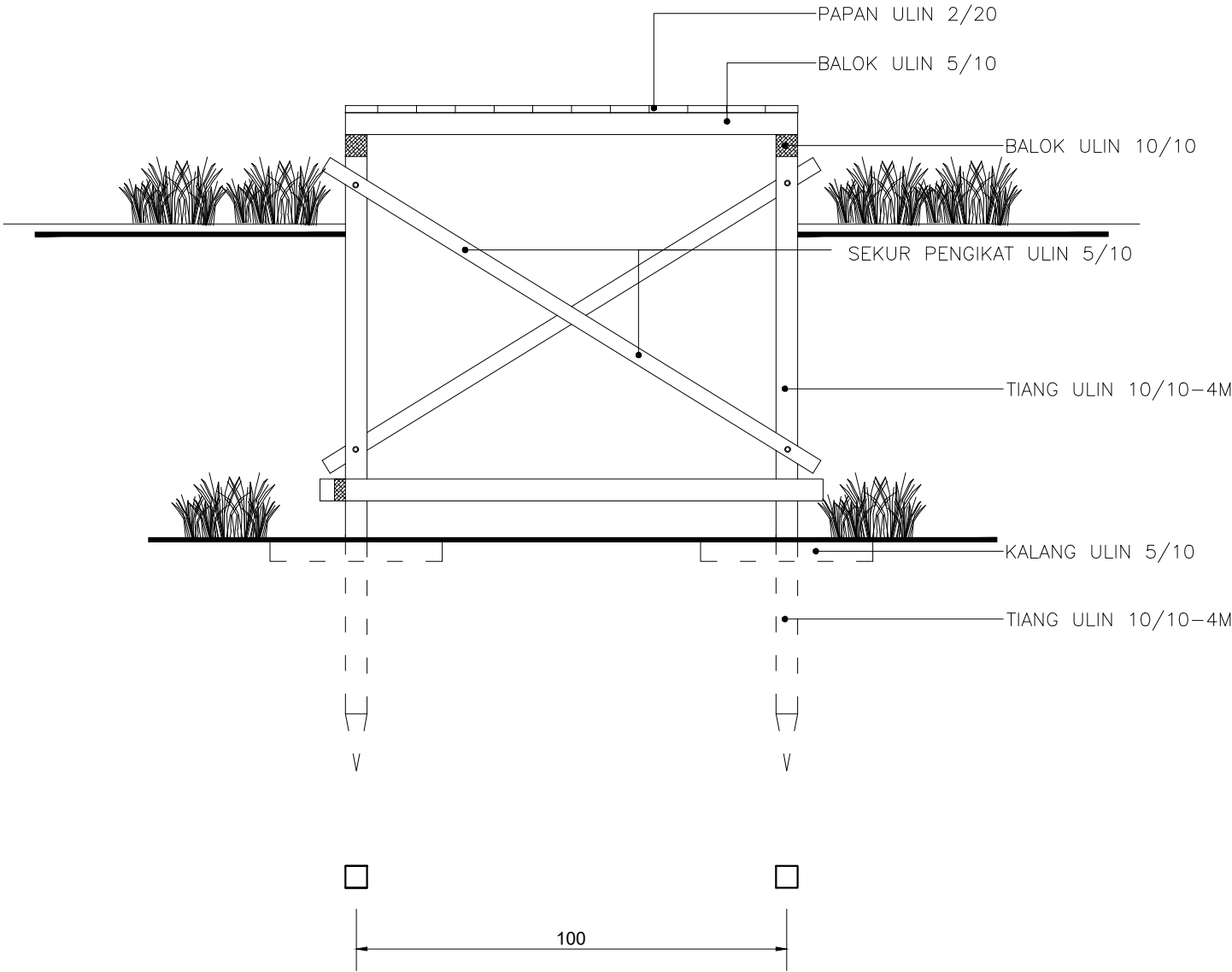
POTONGAN MELINTANG 1 SKALA 1 : 100
